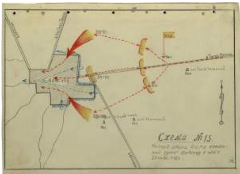
Схема атаки 9-й гв. КД противника в с. Каясула в ночь на 30.11.1942 г.
