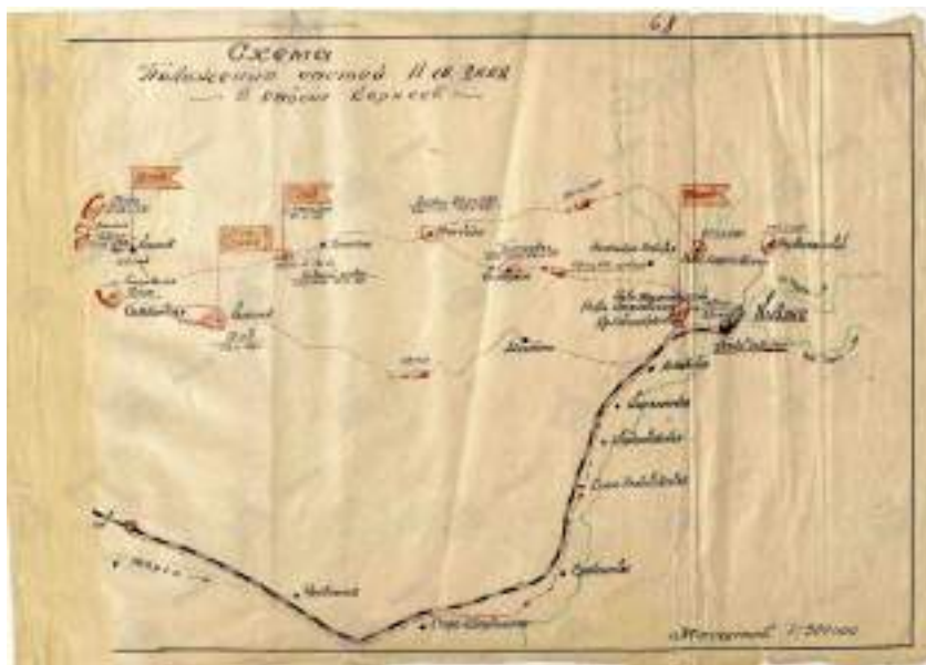
Положение частей 11-й гвардейской кавалерийской дивизии в районе хутора Корнеев
