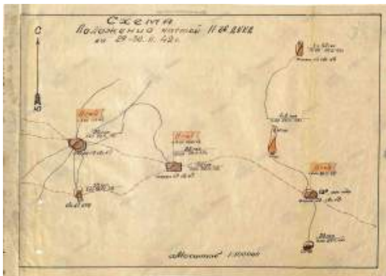
Схема положения частей 11-й гв. КД на 29–30.11.1942 г.
