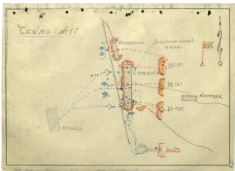
Отход 9-й гв. КД от н.п. Сунженский и положение частей на 19.12.1942 г.
