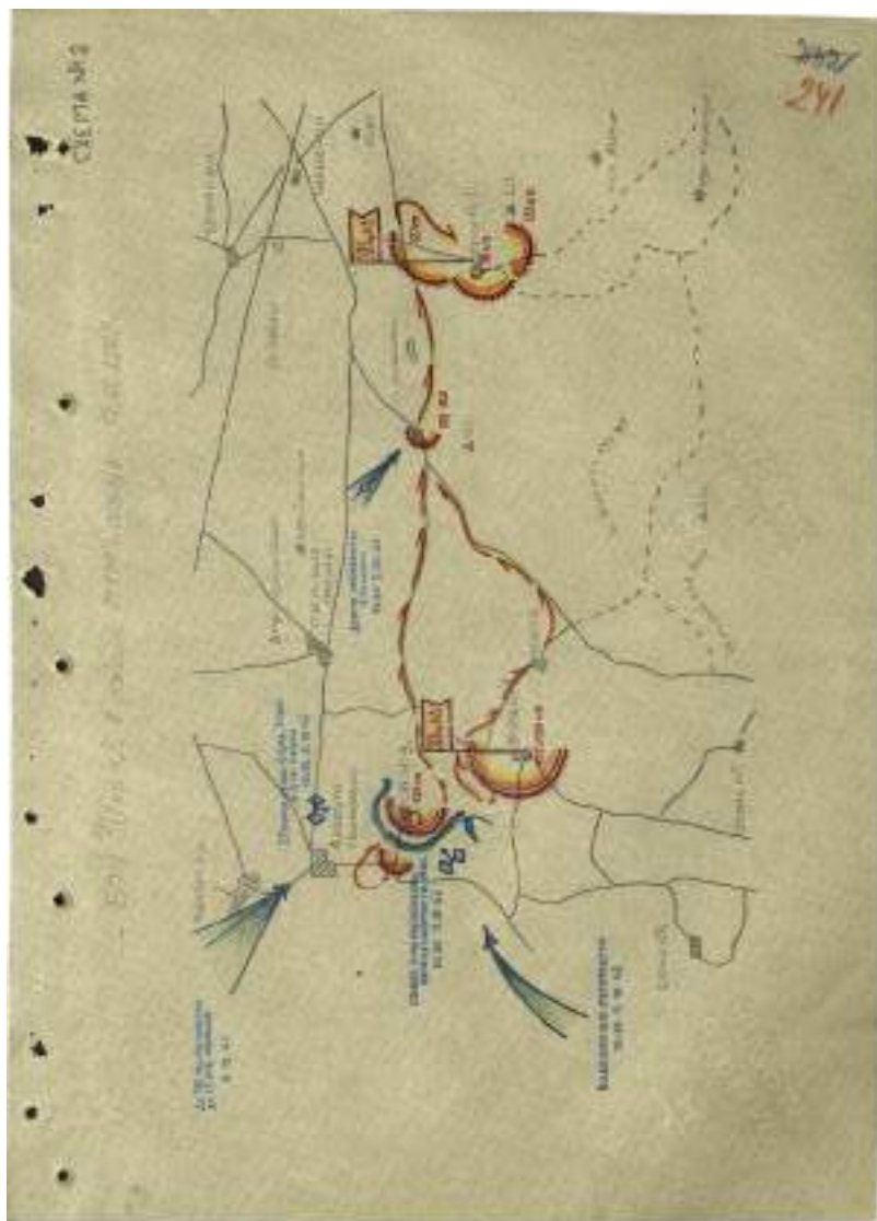
Схема боя 30-й КД в районе МТМ и совхоза № 8 4.10.1942 г.
